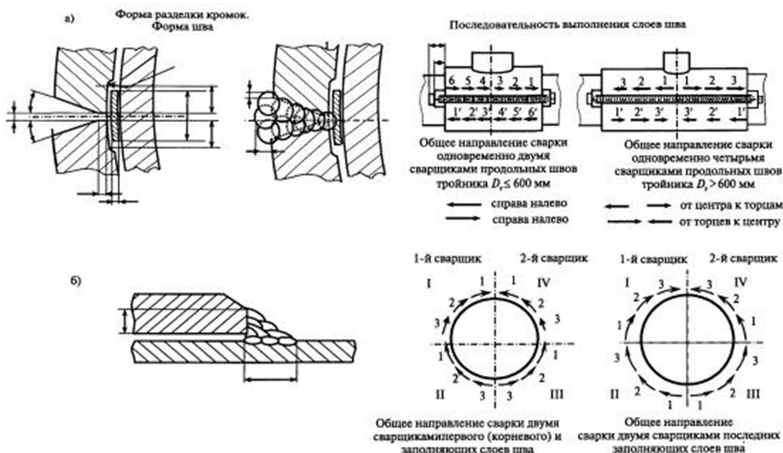
Подготовка под сварку, последовательность сварки, параметры сварного шва
