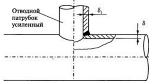
Тип Ia – отводной патрубок усиленный, без накладки
