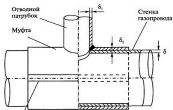
Тип II – разрезная муфта с отводным патрубком
