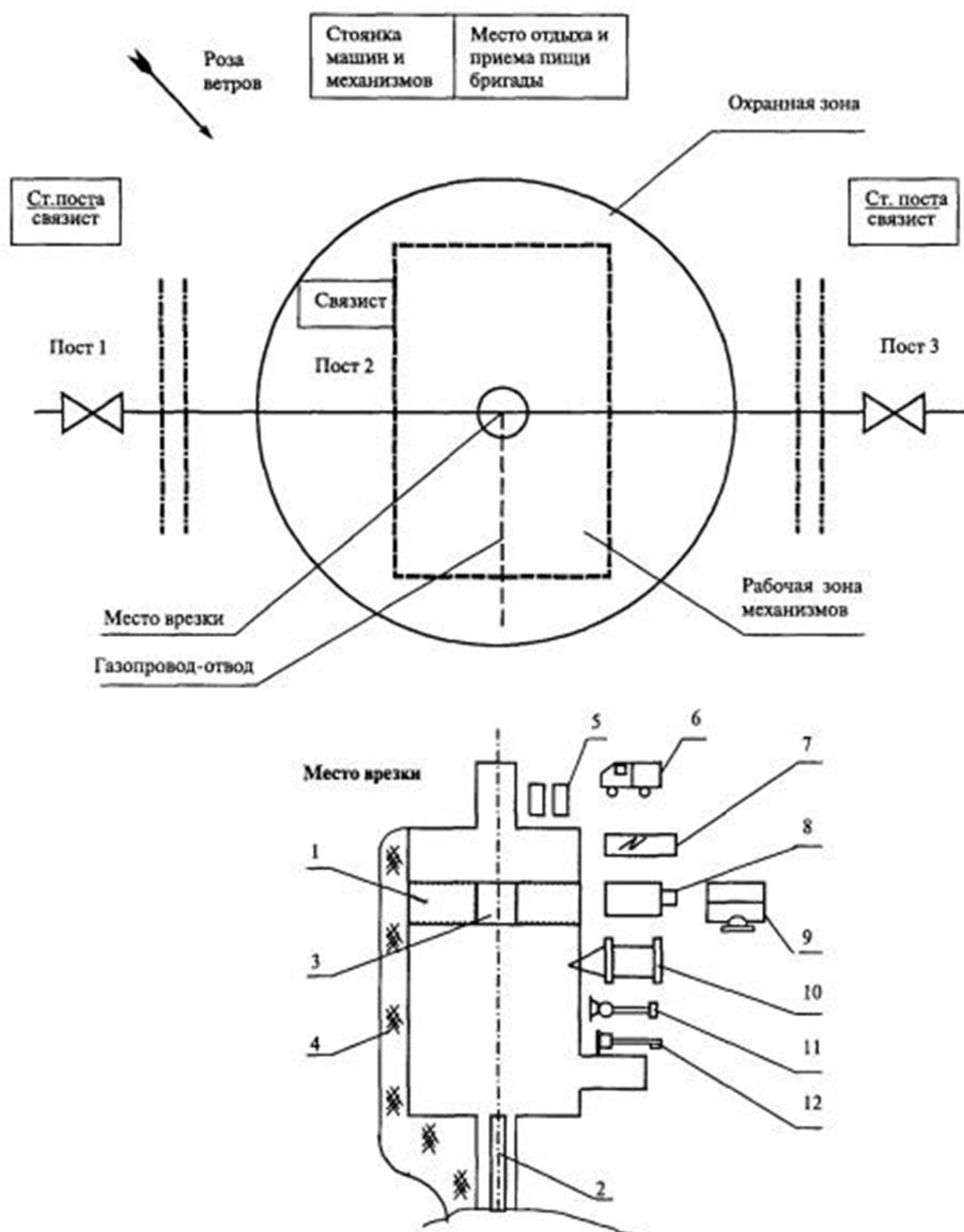
Рисунок 2 - Виды ремонта (замены) участка газопровода, ЗРА, СДТ
