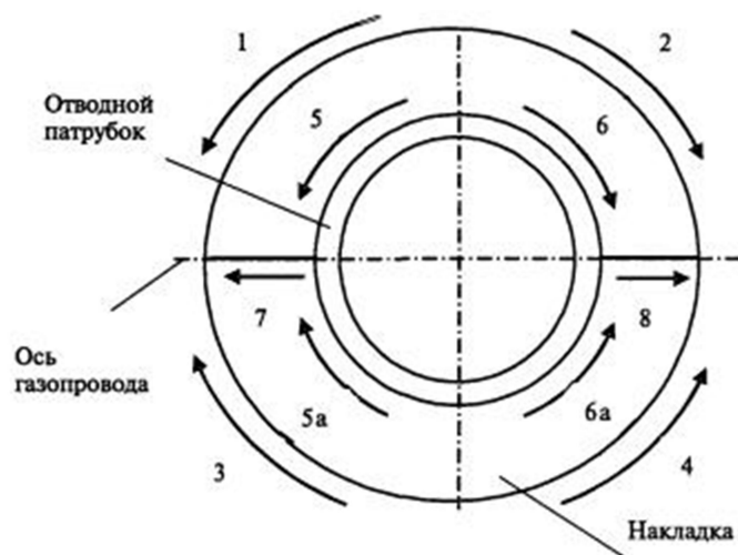
При вертикальной врезке
