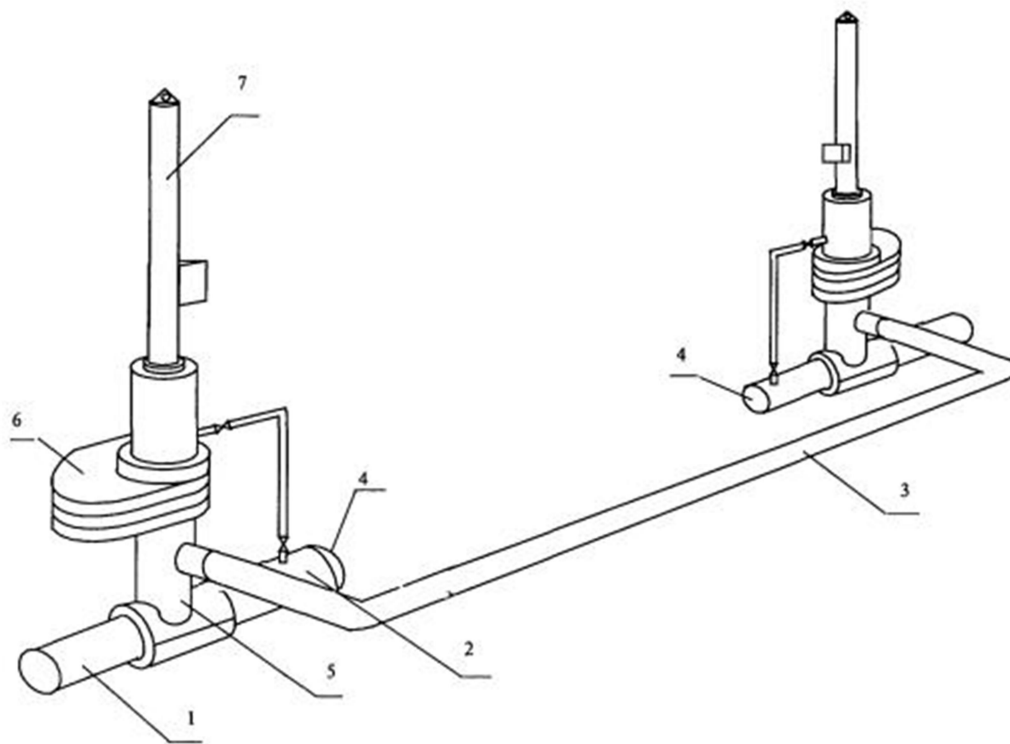
1 - магистральный газопровод; 2 - ремонтируемый участок; 3 - вновь построенный участок газопровода; 4 - сферические заглушки; 5 - разрезной тройник с боковым ответвлением (тип V); 6 - плоская задвижка запорного устройства; 7 - запорное устройство «Стопл»
