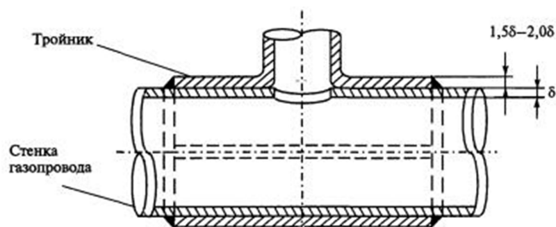
Рисунок 7 - Конструктивное исполнение узла врезки
