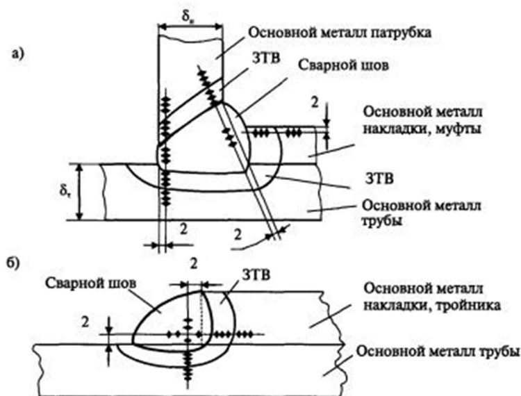
а - угловое соединение конструкций типов I, II; б - угловое (нахлесточное) соединение конструкций типов I, III, IV, V
