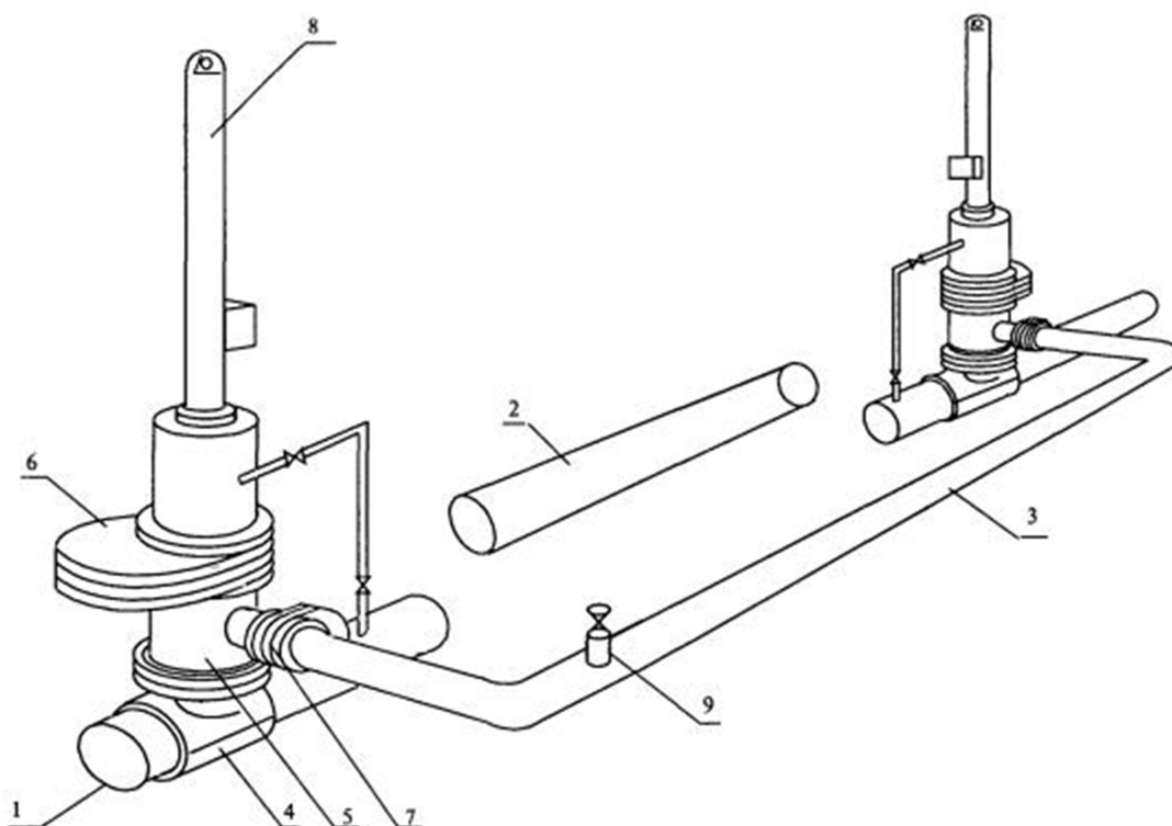
1 - магистральный газопровод; 2 - ремонтируемый участок; 3 - байпас; 4 - разрезной тройник запорного устройства (тип III, IV); 5 - фланцевый адаптер с боковым ответвлением; 6 - плоская задвижка запорного устройства; 7 - плоская задвижка временного байпаса; 8 - запорное устройство; 9 - свеча временного байпаса
