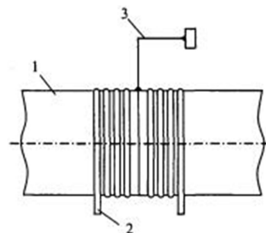
Рисунок Г.7.6 - Схема крепления горячего спая термопары
