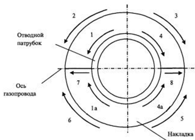
При вертикальной врезке
