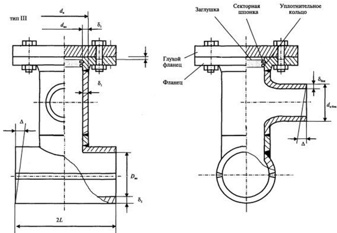
Рисунок В.4 - Тройник разрезной сварной с боковым ответвлением в комплекте с заглушкой и глухим фланцем
