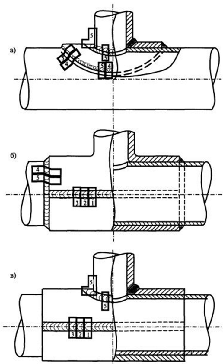
а) конструкций типа I; б) конструкций типов III, IV, V; в) конструкций типа II
