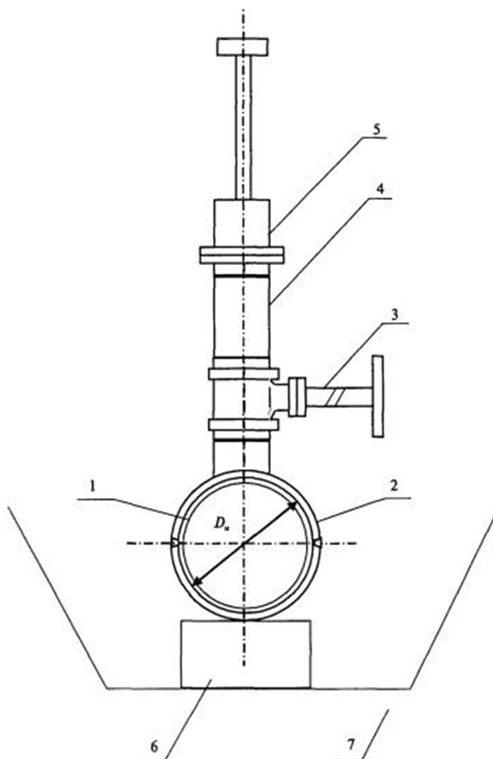
1 - магистральный газопровод с наружным диаметром D_n ; 2 - узел врезки типов I-IV; 3 - шаровой кран; 4 - переходной патрубок; 5 - машина для врезки; 6 - фундаментная плита под узел врезки; 7 - котлован
