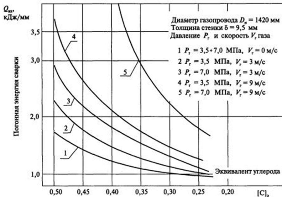
Рисунок Д.7 - Определение погонной энергии приварки узла врезки на газопроводе D 1420 \times 9,5 под давлением
