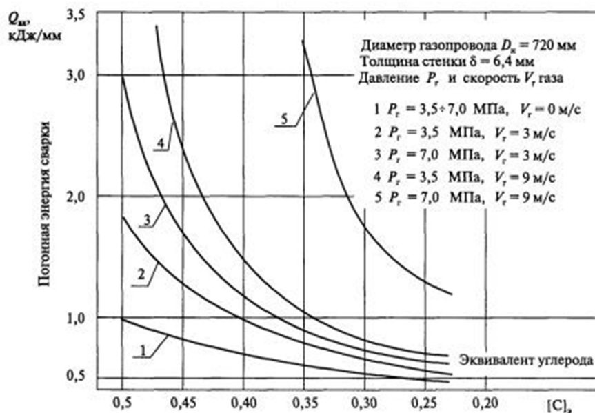
Рисунок Д.2 - Определение погонной энергии приварки узла врезки на газопроводе D 720 \times 6,4 мм под давлением
