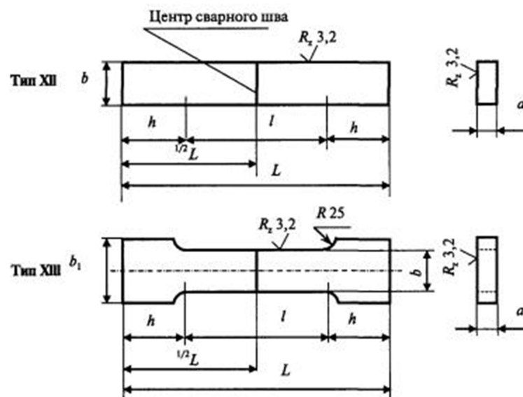
Рисунок Г.3.3 - Форма и размеры образцов (типы XII и XIII) для испытаний сварного соединения на статическое растяжение
