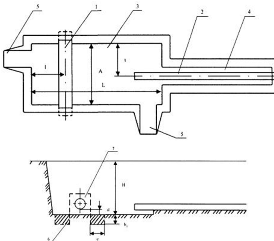
1 - магистральный газопровод; 2 - газопровод-отвод; 3 - котлован; 4 – траншея газопровода-отвода; 5 - выход из котлована; 6 - «карман» с насыпным грунтом; 7 - контур грунта, разрабатываемого вокруг трубы вручную
