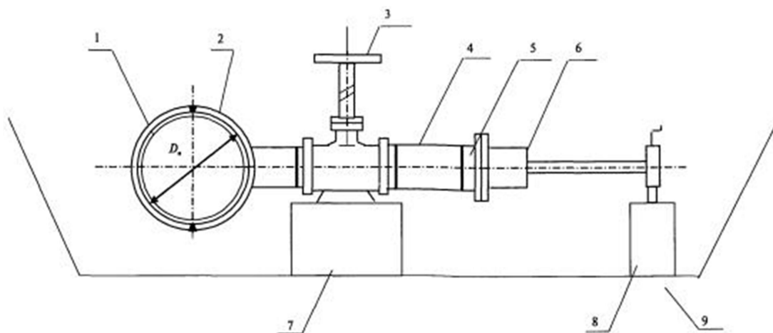
1 - магистральный газопровод с наружным диаметром D_n ; 2 - узел врезки типов I-IV с концом ответвления под приварку; 3 - шаровой кран; 4 - переходной патрубок; 5 - ответный фланец; 6 - машина для врезки; 7 - фундаментная плита под шаровой кран; 8 - опора под машину для врезки; 9 - котлован
