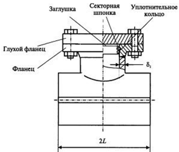
Рисунок В.3 - Тройник разрезной сварной, штамповарной (типы III, IV) во фланцевом исполнении в комплекте с заглушкой и глухим фланцем
