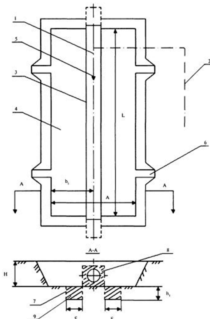
1 - ось магистрального газопровода; 2 - ось байпаса; 3 - магистральный газопровод; 4 - котлован; 5 - направление транспорта газа; 6 - выход из котлована; 7 - «карманы»; 8 - грунт, разрабатываемый вокруг трубы вручную; 9 - насыпной грунт
