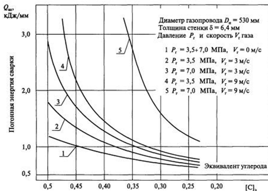
Рисунок Д.1 - Определение погонной энергии приварки узла врезки на газопроводе D 530 \times 6,4 мм под давлением
