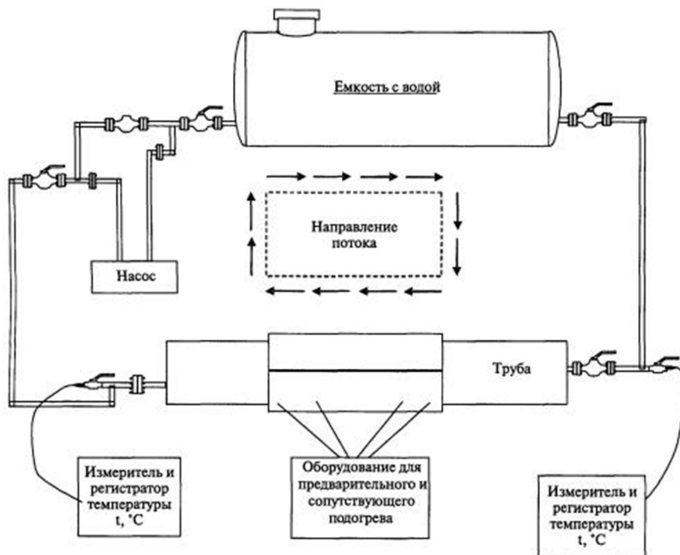
Рисунок Г.1.1 - Типовая схема стенда для производственной аттестации технологий сварки узлов врезки в конденсатопровод
