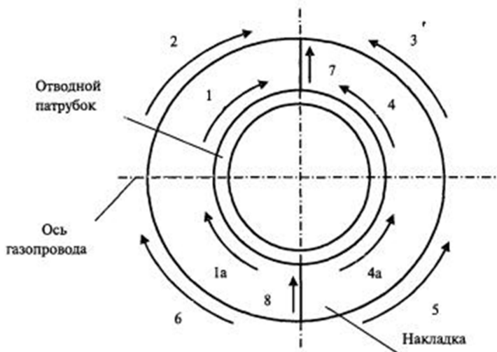
При горизонтальной врезке
