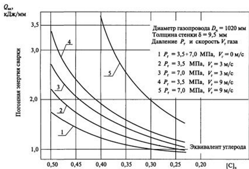
Рисунок Д.5 - Определение погонной энергии приварки узла врезки на газопроводе D 1020 \times 9,5 \text{ мм} под давлением
