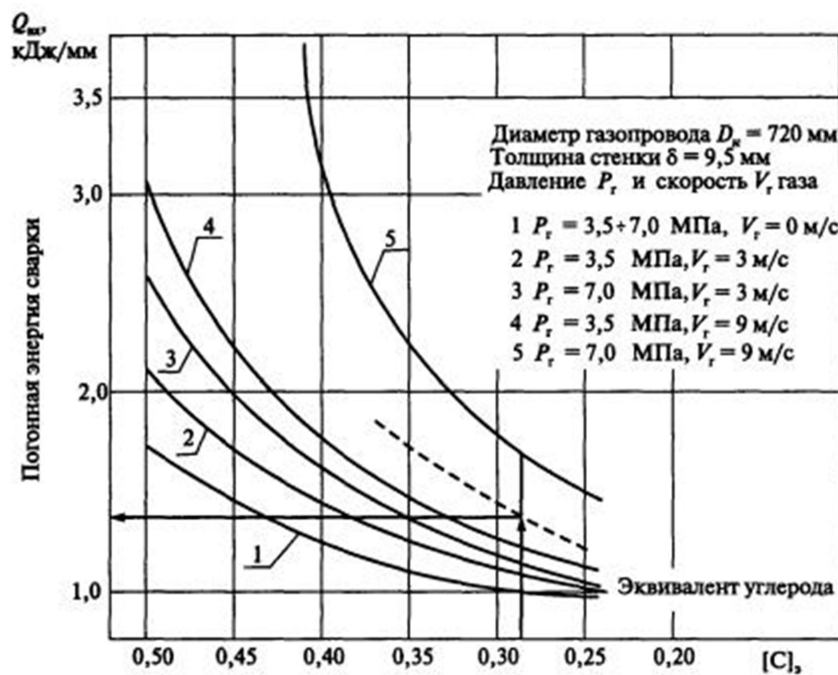
Рисунок Д.4 - Определение погонной энергии приварки узла врезки на газопроводе D 720 \times 9,5 мм под давлением
