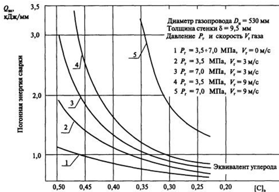
Рисунок Д.3 - Определение погонной энергии приварки узла врезки на газопроводе D 530 \times 9,5 мм под давлением
