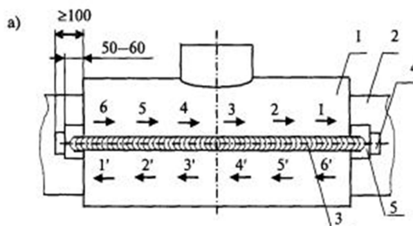
Рисунок 14 - Последовательность наложения слоев при сварке продольных швов разрезного тройника
