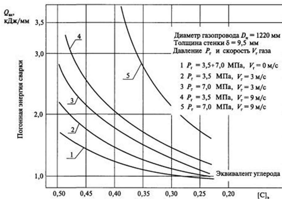
Рисунок Д.6 - Определение погонной энергии приварки узла врезки на газопроводе D 1220 \times 9,5 \text{ мм} под давлением
