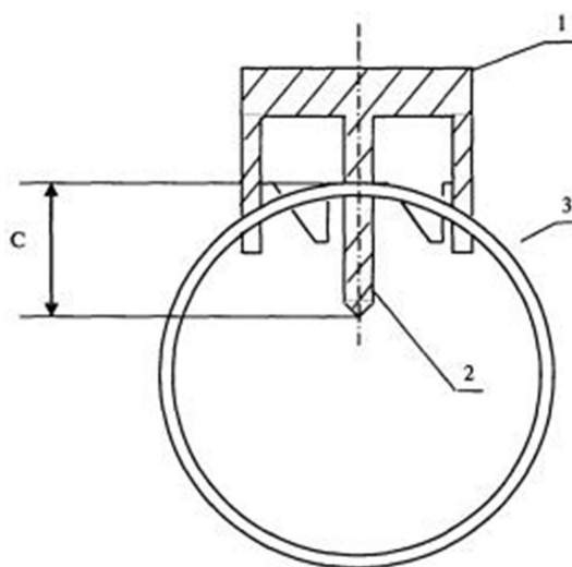
Рисунок Е.1 - Конструктивное исполнение ребер жесткости (пример)
