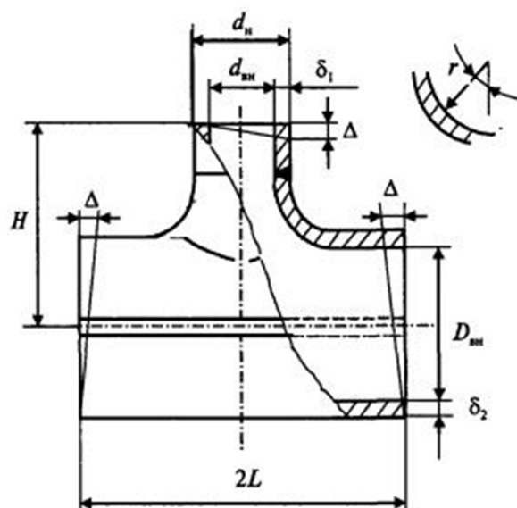
Рисунок В.1 - Тройник разрезной штамповарной
