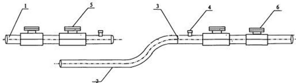
б) вновь построенный участок газопровода (лупинг) с возможностью пропуска устройств очистки и ВТД (пример)
