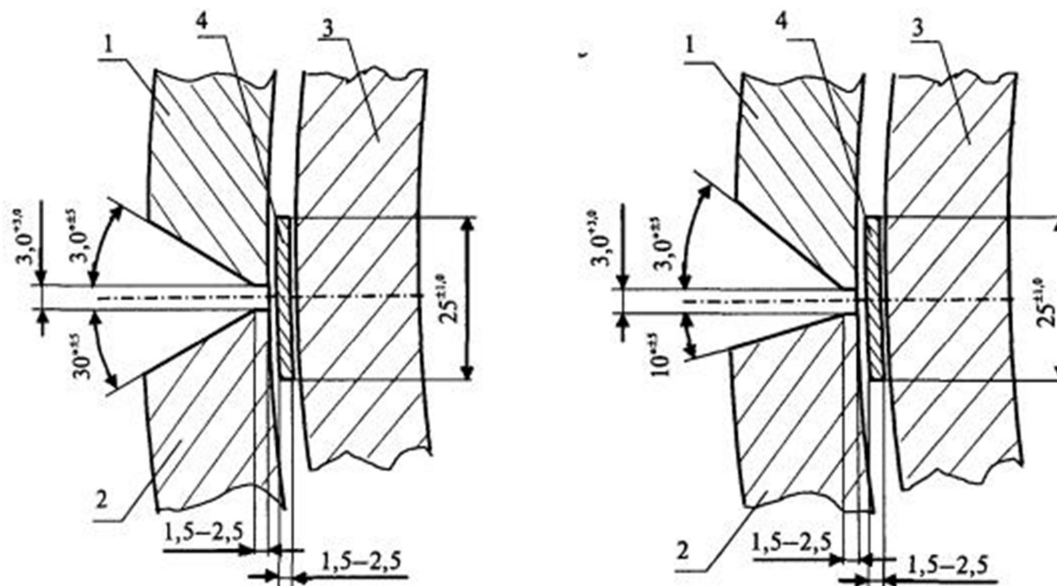
а) с выборкой под подкладную пластину (для тройников - типы III-V и муфт - тип II)
