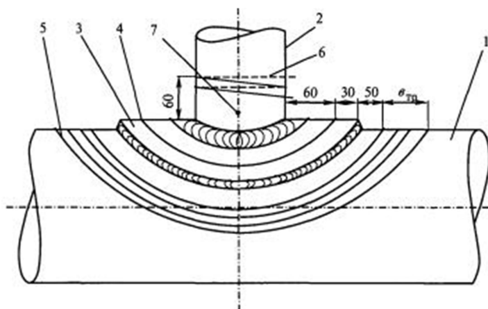
Рисунок Г.7.3 - Схема установки электронагревателей комбинированного действия для нагрева кольцевых нахлесточных сварных соединений накладке с газопроводом
