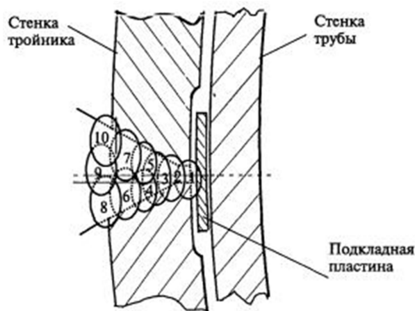
1-10 - порядковые номера слоев приварки тройника
