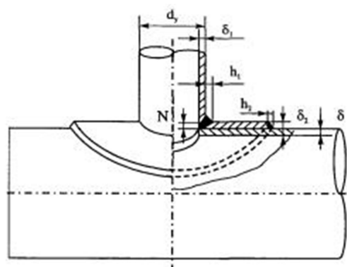
Тип I – отводной патрубок с накладкой
