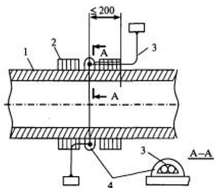
Рисунок Г.7.6 - Схема крепления горячего спая термопары
