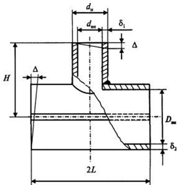
Рисунок В.2 - Тройник разрезной сварной
