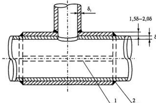
Тип IV – разрезной тройник сварной
